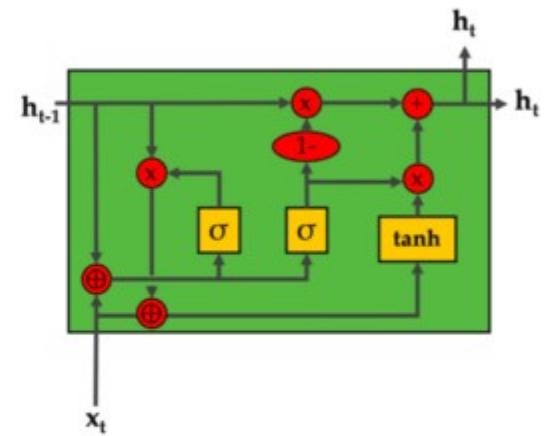
GRU
